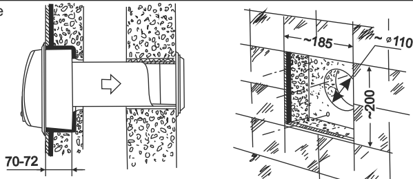
Unterputzmontage in eine blinde Aussparung
