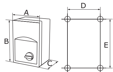
Außenabmessungen, mm
