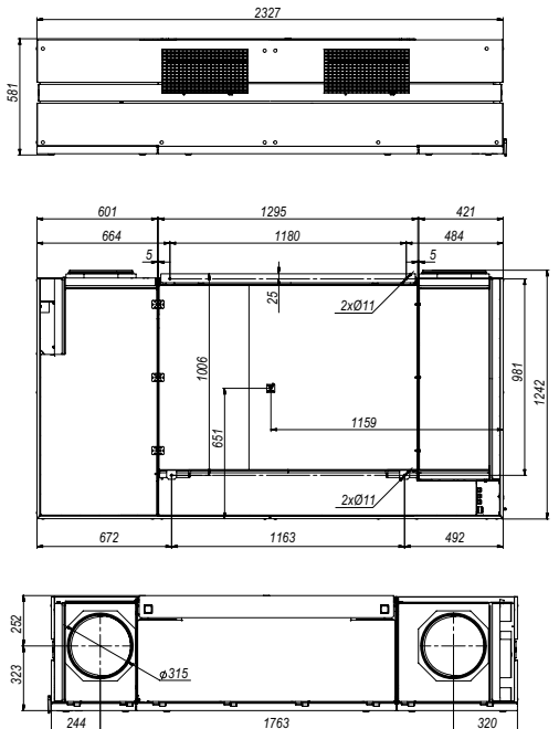
Außenabmessungen für DVUT 1000 PB EC V.2, mm
