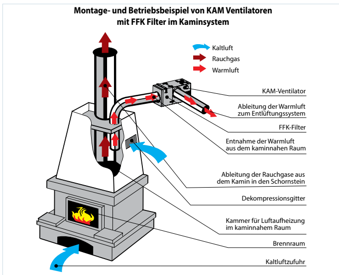
Montage- und Betriebsbeispiel von KAM Ventilatoren mit KFK Rückschlagklappe und KAM Ventilatoren mit der Klappe KFK und GFK (BYPASS) im Kaminsystem
