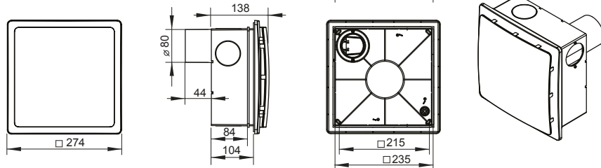
VNV-1 80 KV2
