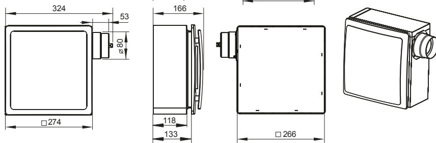
VN-1 80 KP
