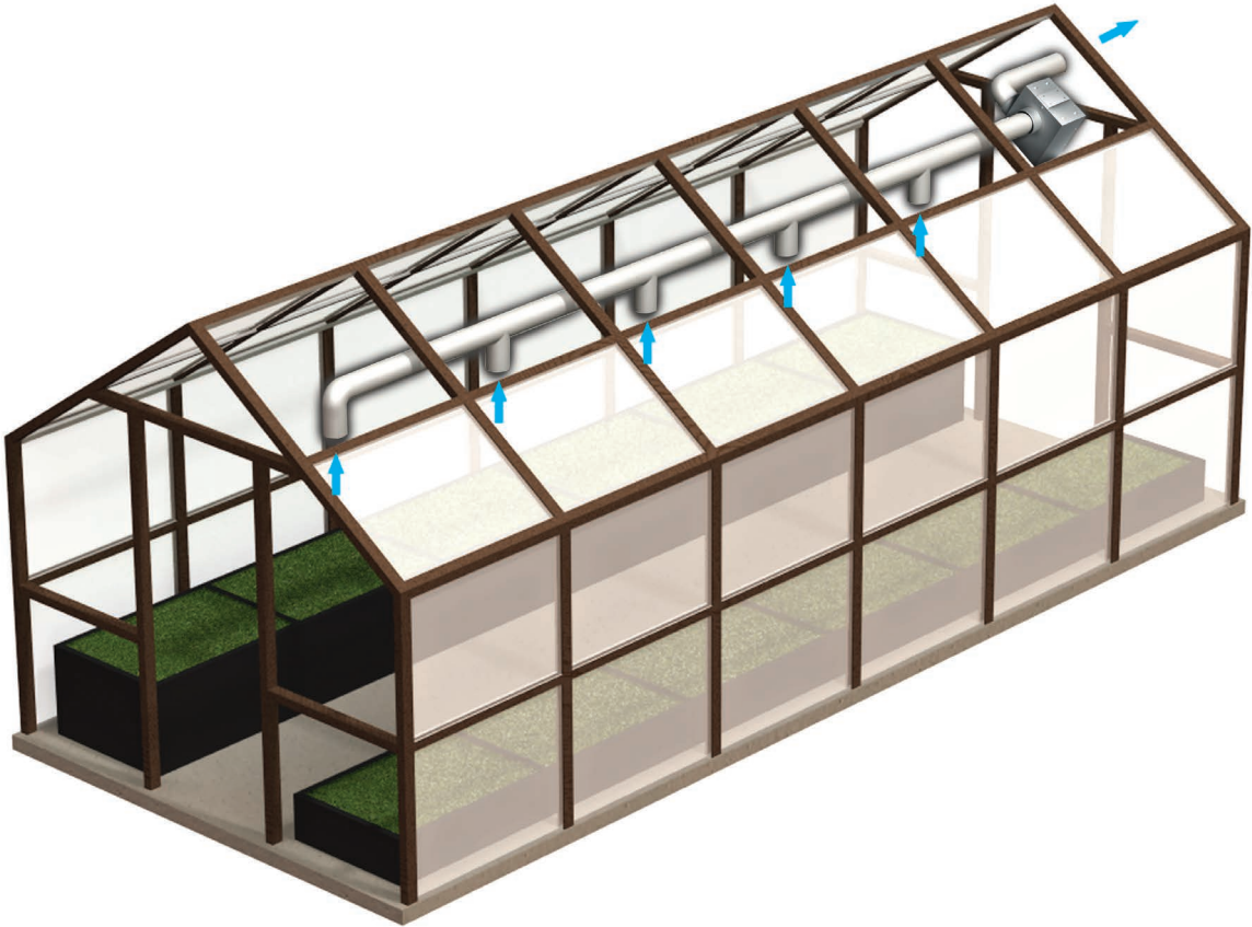
KSA fan greenhouse ventilation example
