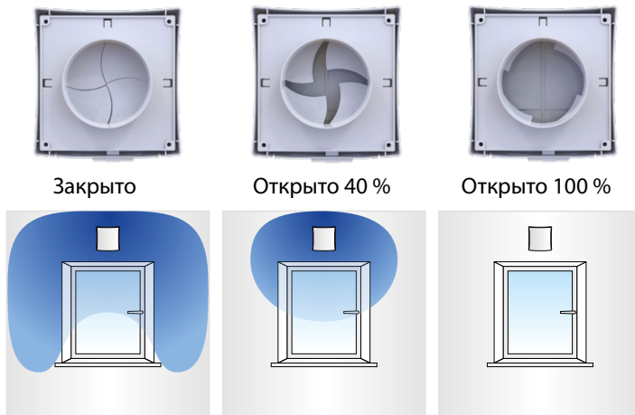
Распределение воздушного потока при различном положении регулятора воздуха
