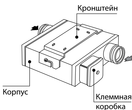
1 вход – 1 выход
