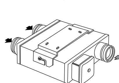
c) ВКП 80..100/80..100 x 2 мини ВКП 125..150/100..125 x 2
