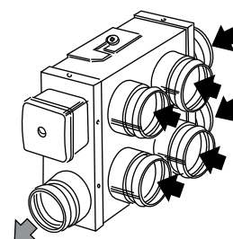
6 входов – 1 выход
