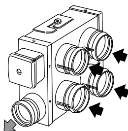
4 входа – 1 выход
