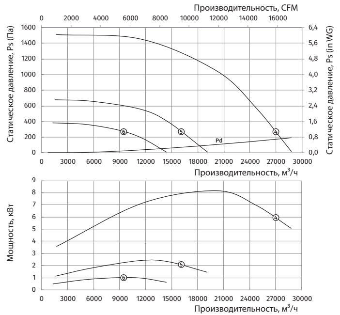
Типоразмер: 710
