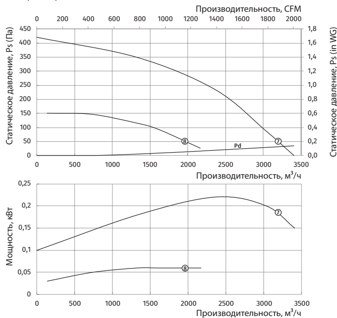
Типоразмер: 355
