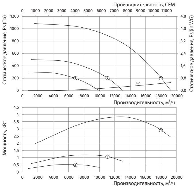
Типоразмер: 630
