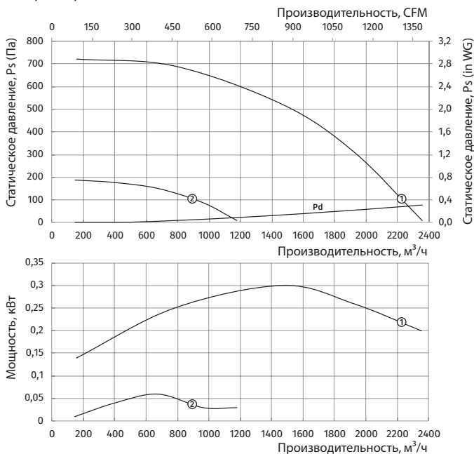
Типоразмер: 250
