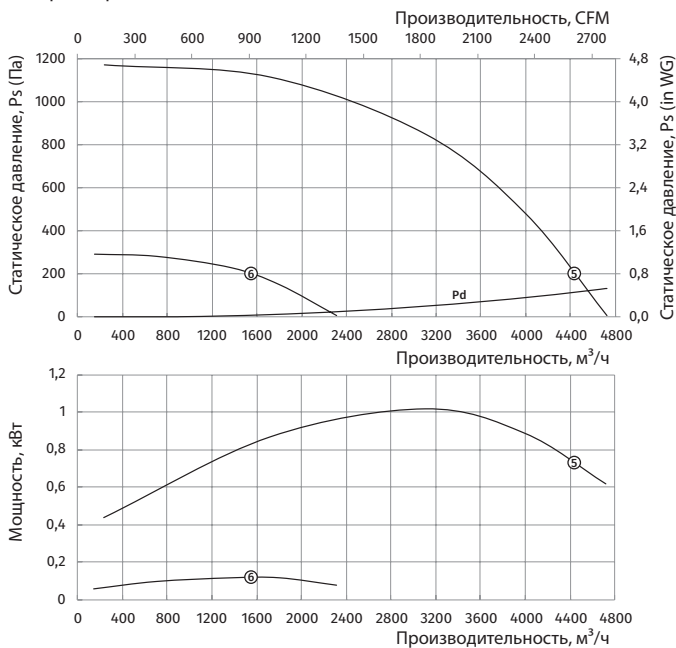
Типоразмер: 315
