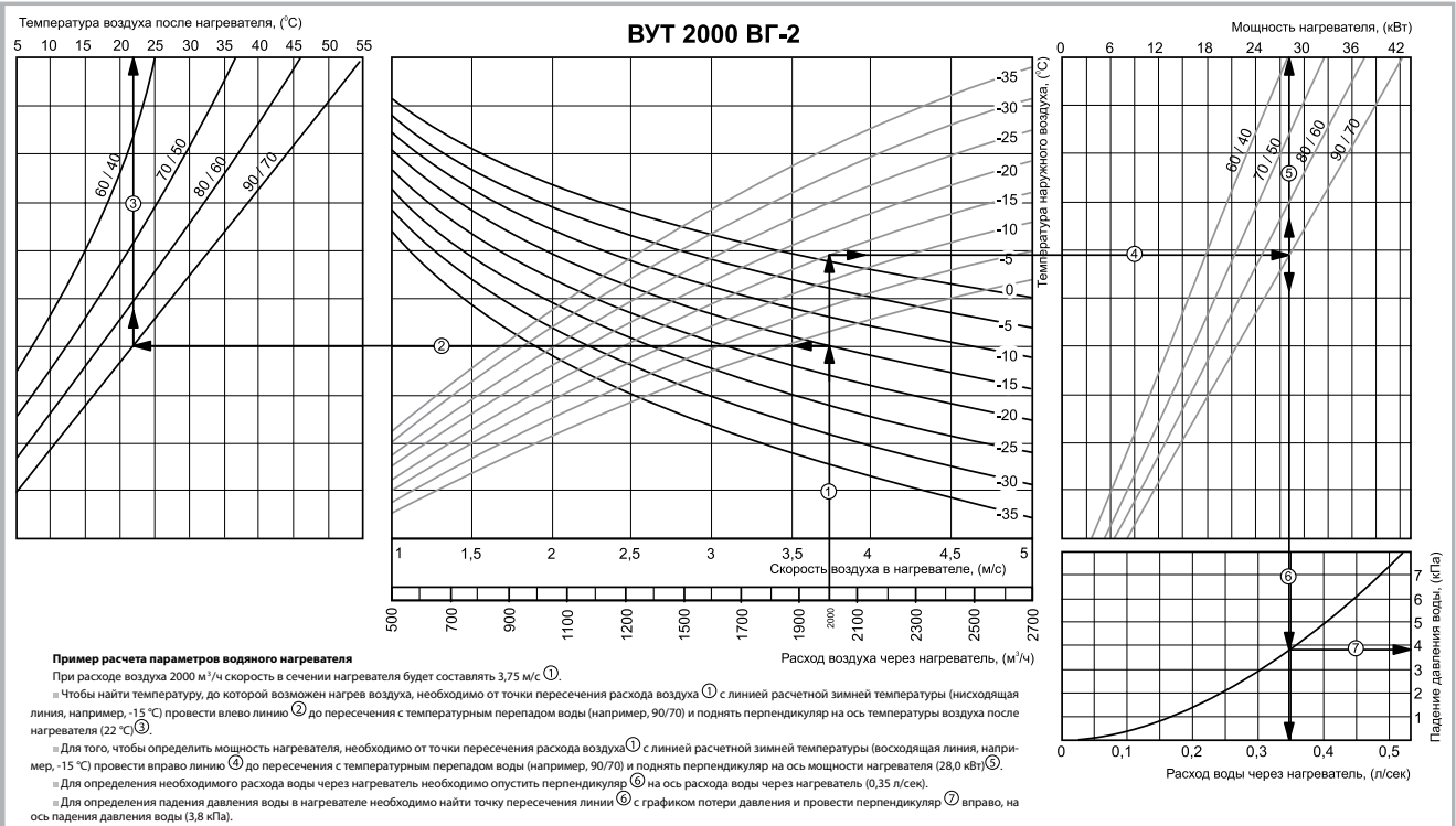
Рис. 8. Определение параметров водяного нагревателя для ВУТ 2000 ВГ-2
