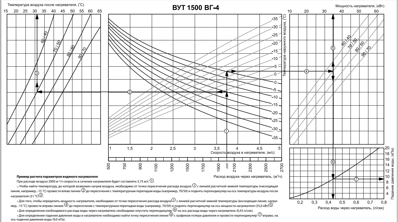
Рис. 7. Определение параметров водяного нагревателя для ВУТ 1500 ВГ-4
