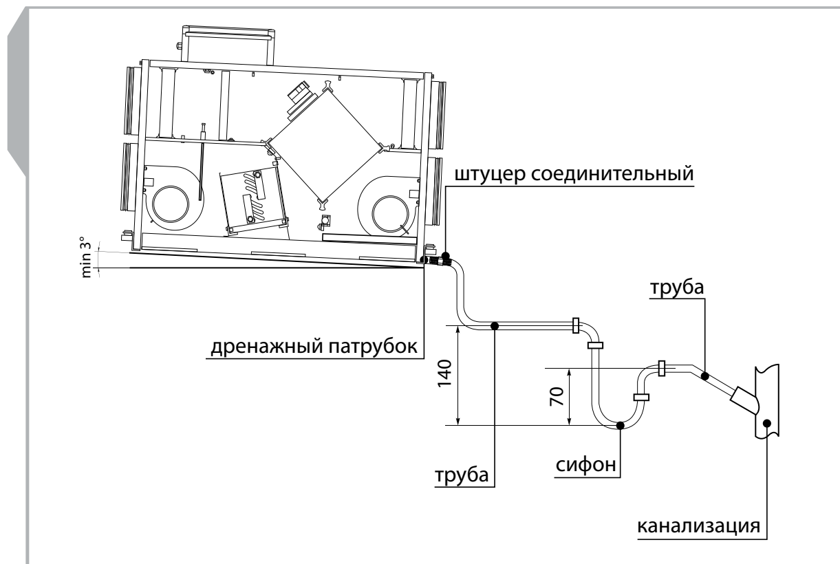
Рис. 15. Отвод конденсата
