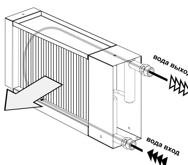
б) противоточное подключение
