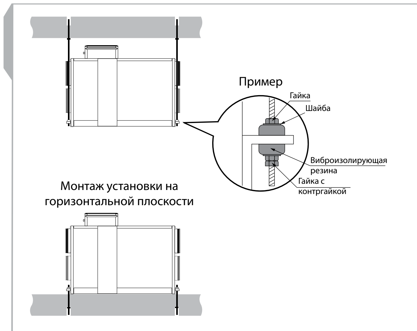
Рис. 11. Монтаж установки
