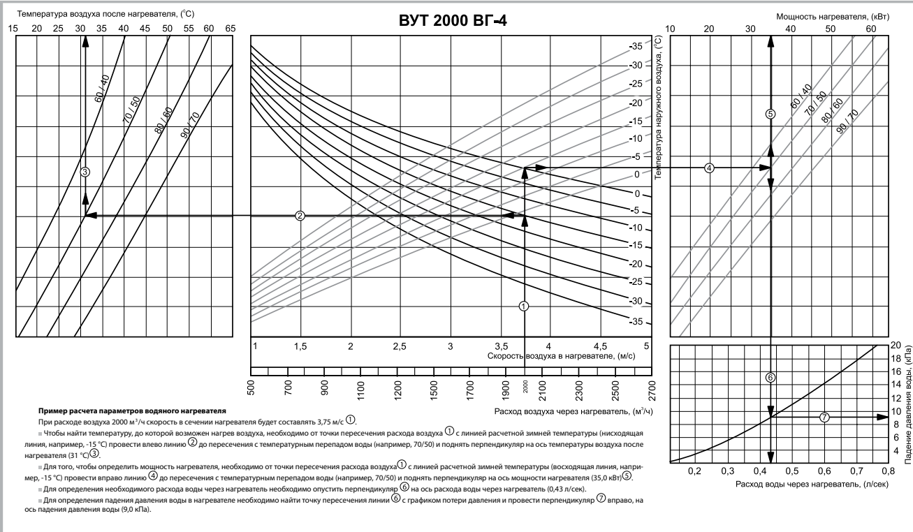
Рис. 9. Определение параметров водяного нагревателя для ВУТ 2000 ВГ-4
