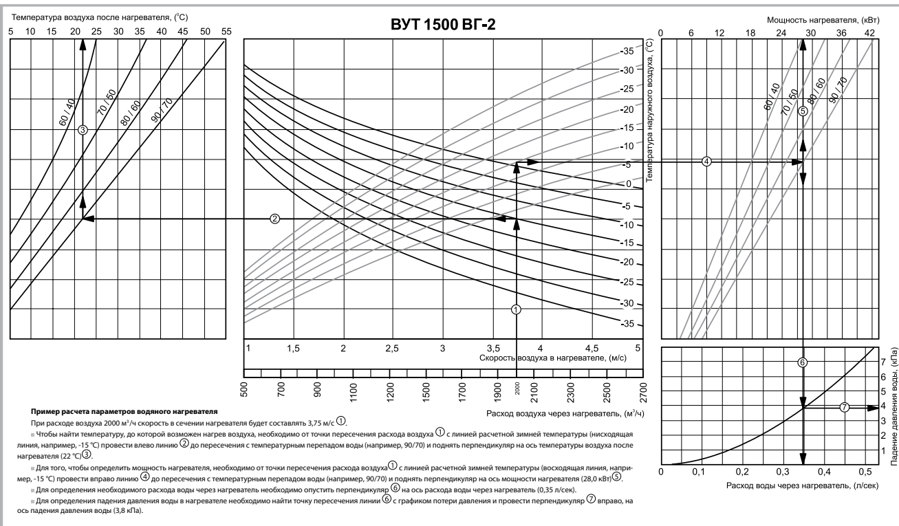
Рис. 6. Определение параметров водяного нагревателя для ВУТ 1500 ВГ-2
