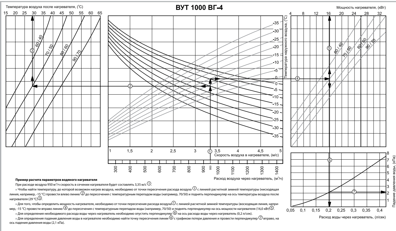
Рис. 5. Определение параметров водяного нагревателя для ВУТ 1000 ВГ-4
