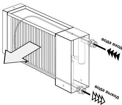
а) прямоточное подключение
