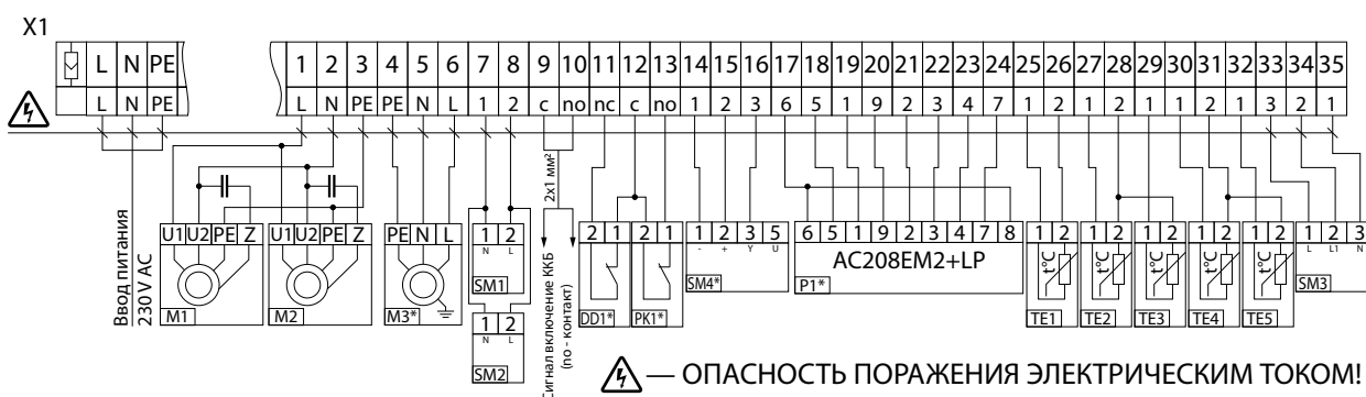
Рис. 17. Схема внешних подключений ВУТ 800 (1000) ВГ
