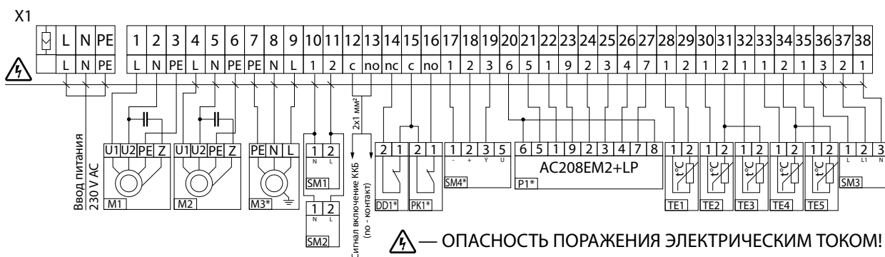
Рис. 18. Схема внешних подключений ВУТ 1500 (2000) ВГ
