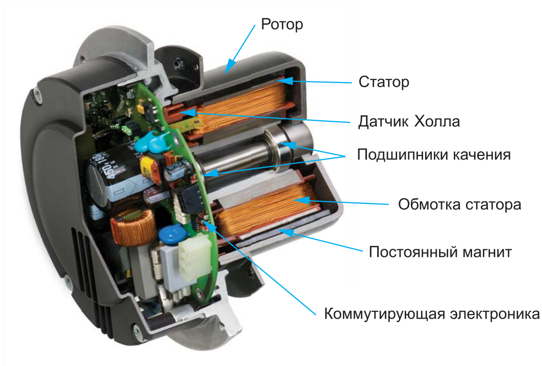
Устройство энергосберегающего ЕС-двигателя
