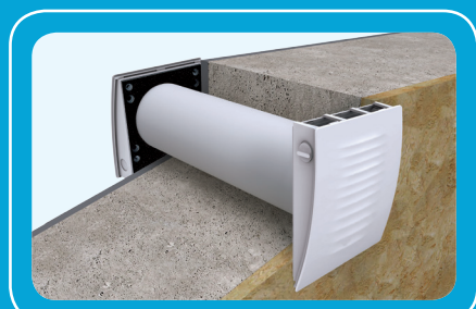
Монтаж в стену стандартной толщины с применением наружной решетки ЕН-14
