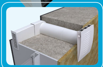
Скрытый монтаж с применением набора для углового монтажа ИП
